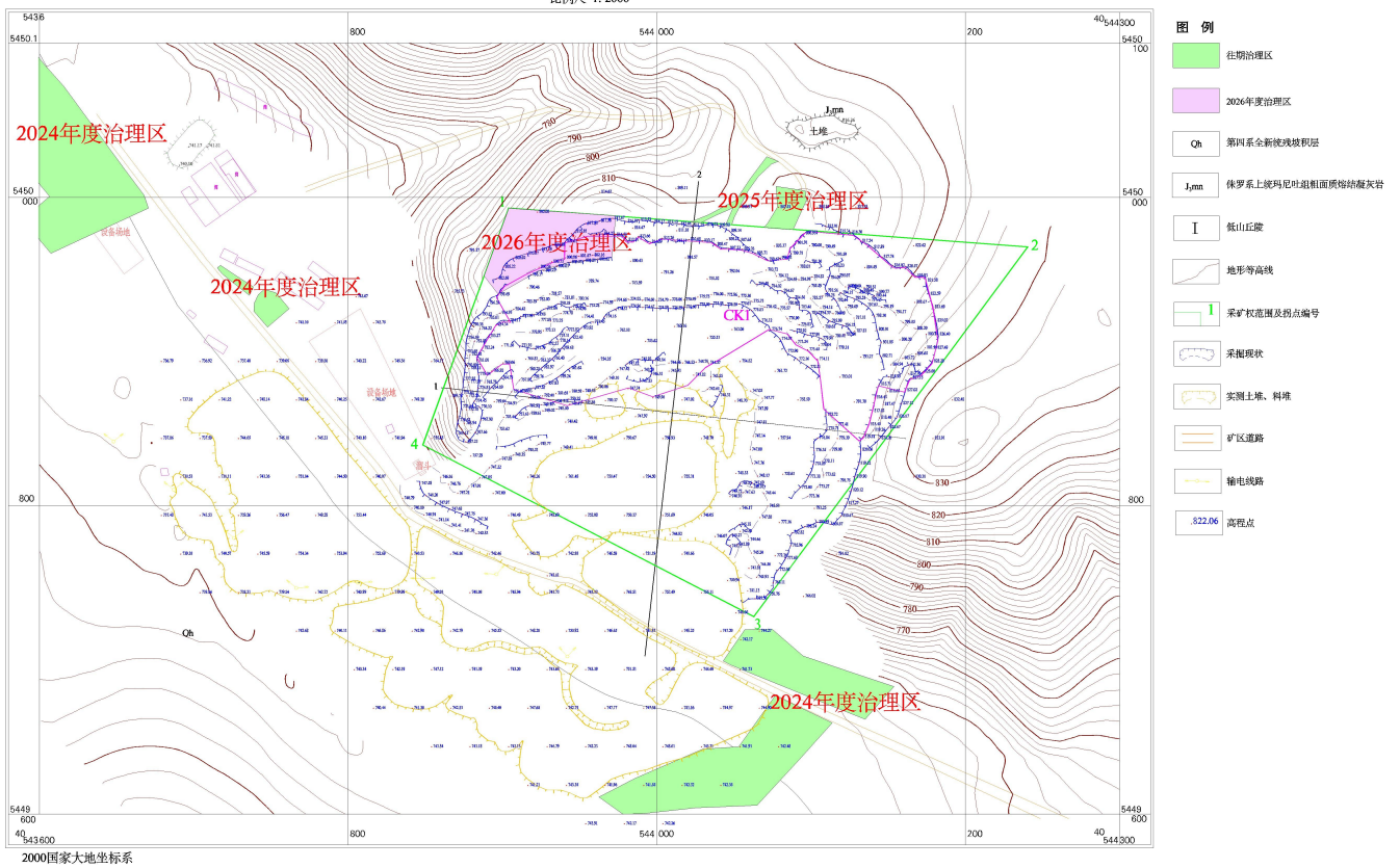
2026年度大雁矿区丰鑫缘采石场矿山地质环境治理与土地复垦工作部署图 比例尺 1:2000
